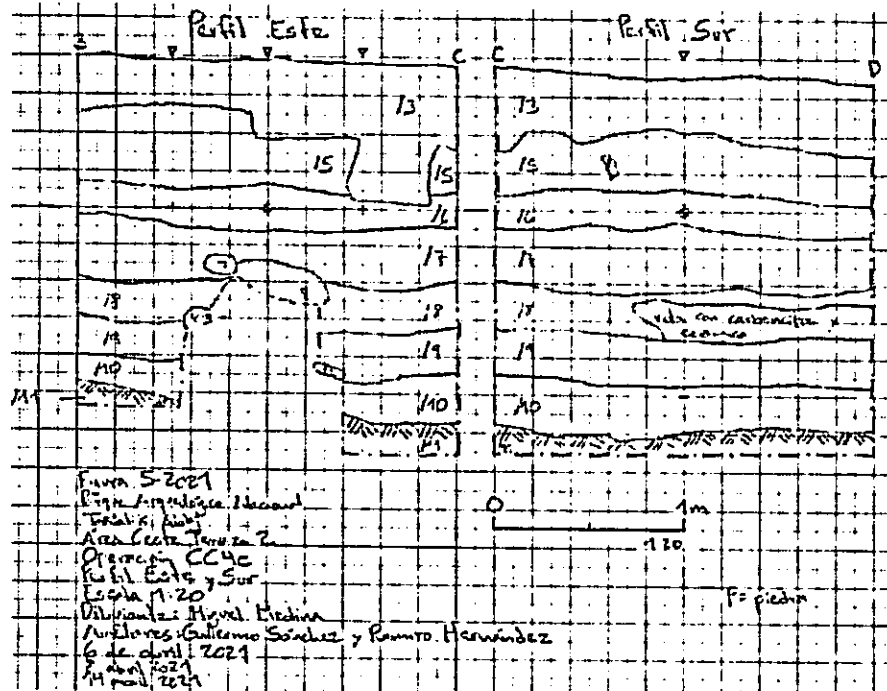
Figura 4. Dibujo de los perfiles este y sur de la Operación CC4c (Parque Arqueológico Nacional Tak'alik Ab'aj, MICUDE-DGPCN/IDAEH 2021).
